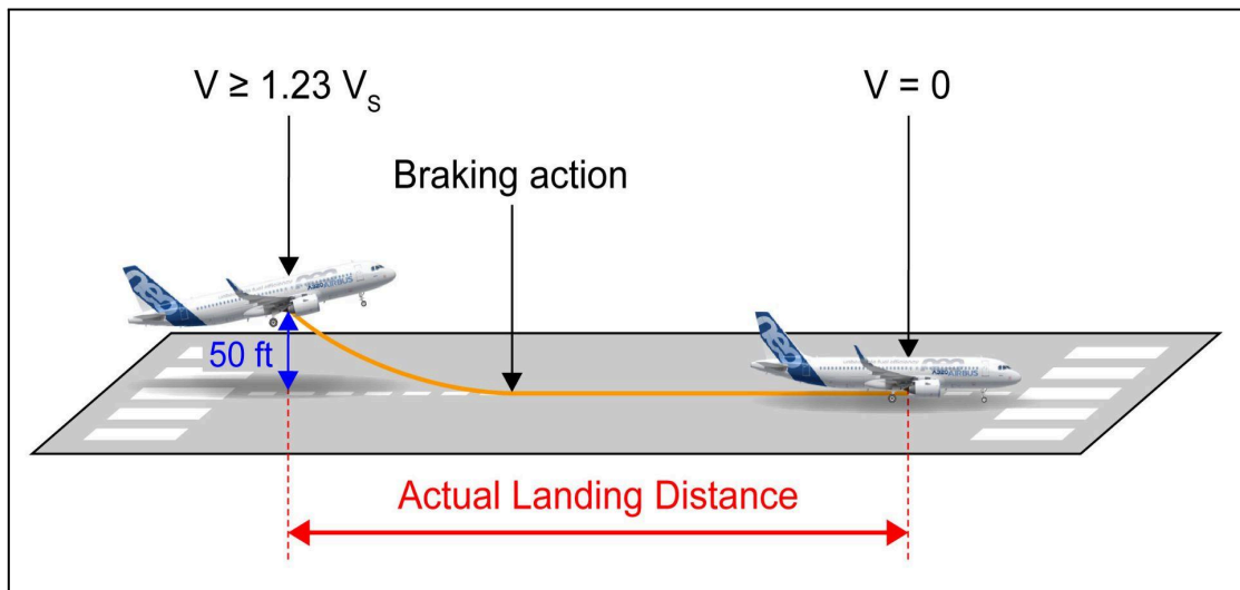
Illustration F-4: Actual Landing Distance
